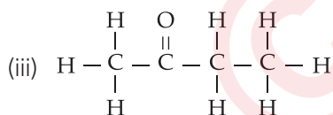
But-2-one
